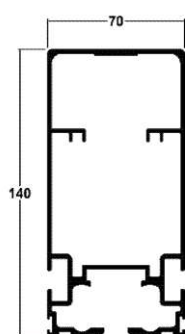
ΠΡΟΦΙΛ ΟΔΗΓΟΥ 70X140 GUIDE PROFILE 70X140
