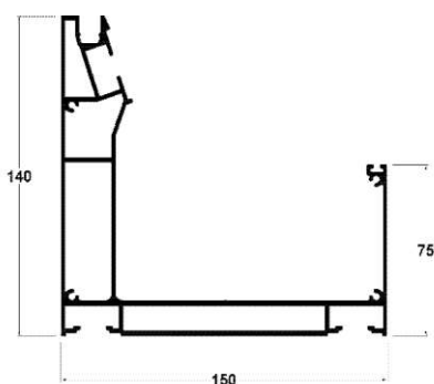
ΠΡΟΦΙΛ ΣΤΗΘΑΙΟΥ-ΥΔΡΟΡΡΗΣΗΣ BEAM-GUTTER FRONT PROFILE
