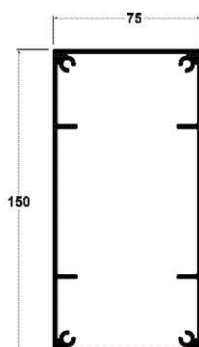
ΠΡΟΦΙΛ ΚΟΛΩΝΑΣ 75X150 PILLAR PROFILE 75X150
