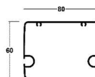
ΑΚΡΙΑΝΟ ΠΡΟΦΙΛ ΠΑΝΙΟΥ TERMINAL BAR PROFILE
